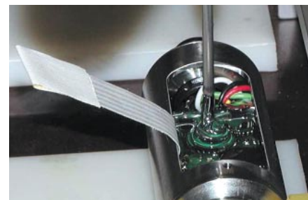
Bild 4. Sensorverguss mit Hochtemperatur-Gel ISO-PUR A 776
